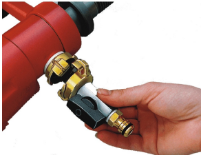
DK09: Kugelhahn ankuppeln bereit zum Nassbohren
